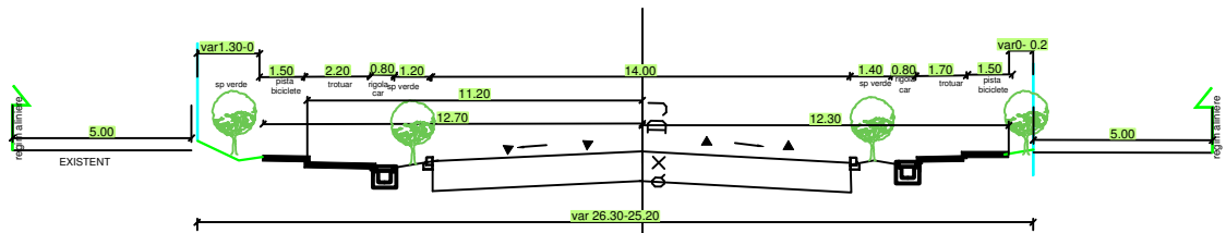
Profil propus 1-1-DJ 101D-asfaltat scara 1:100
